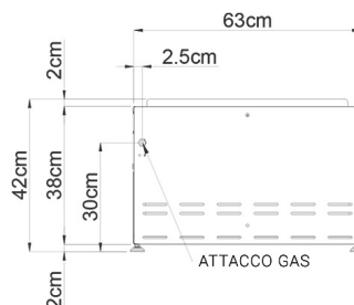
VISTA POSTERIORE
