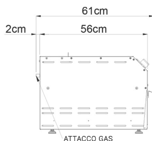
VISTA LATERALE
