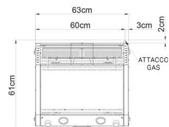
VISTA SUPERIORE
